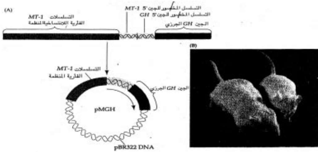
الشكل (15): التقانة الحيوية. (A) مخطط ترسمي لتحضير بناء جيني يتألف من جين هرمون النمو GH الجردي، والتسلسلات المنظمة لجين الميتالوتيونين MT-1، تفرز كلها مع التسلسلين المخوضرين في البلازميد PBR322 للحصول على فأر عملاق (الأيسر في B). (عن المرجع ٢، ص ٤٠٨. انظر المرجع والنص من أجل التفاصيل).
